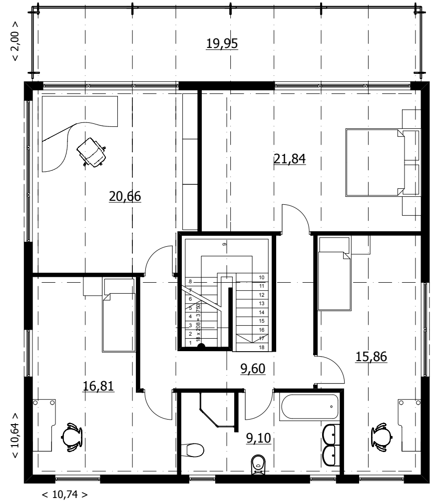
План 2-го этажа на отм. +3,750м (М1:100)
