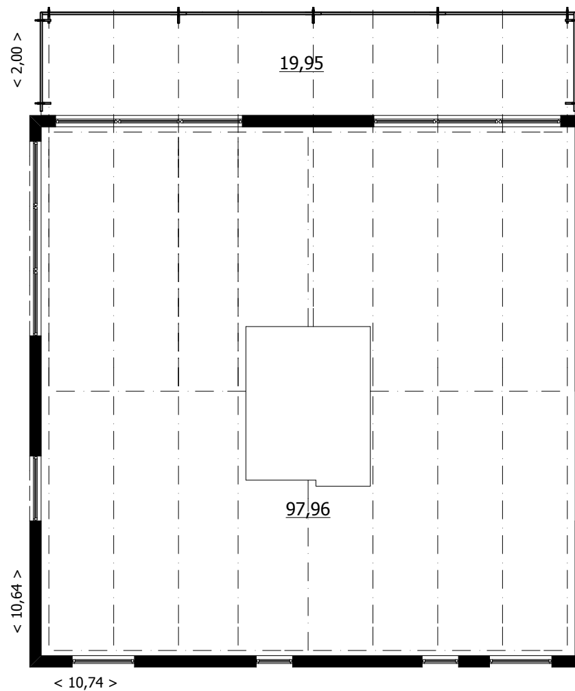
План 2-го этажа на отм. +3,750м (М1:100)
